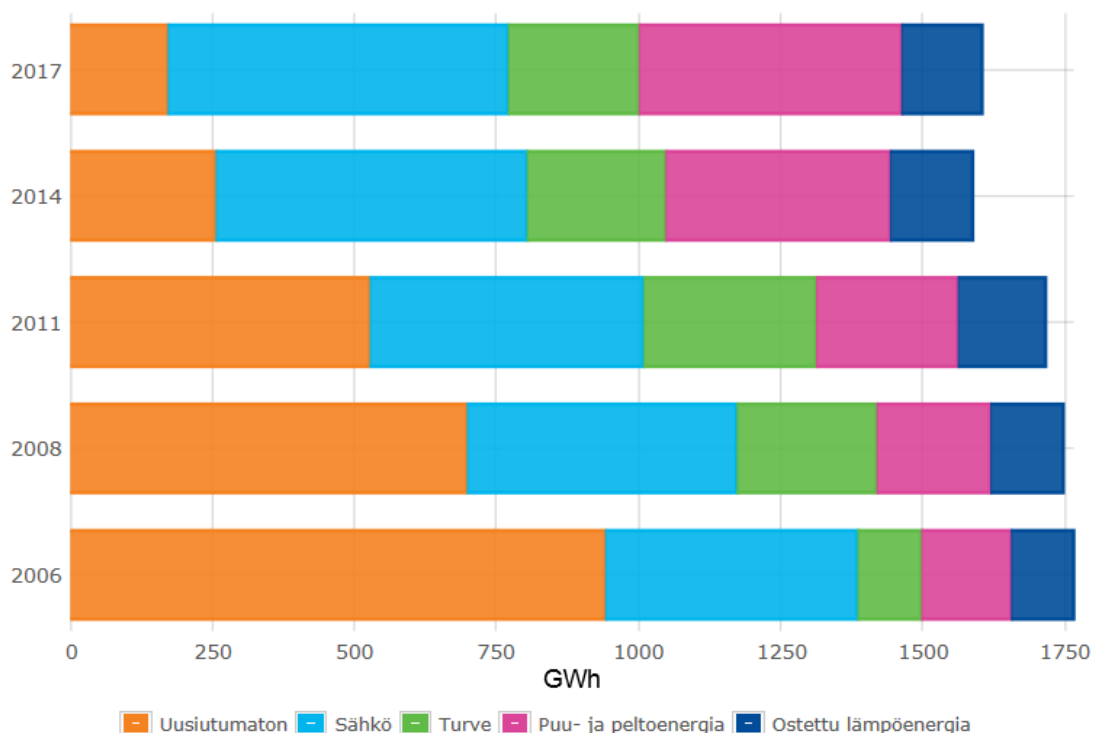
Kuva 5 Kasvihuoneyritysten energiankulutus 2006-2017. Uusiutumaton energia kuvaa tässä fossiilisista energiaa. Sähköenergiaa ei ole laskettu primaarienergiana.
